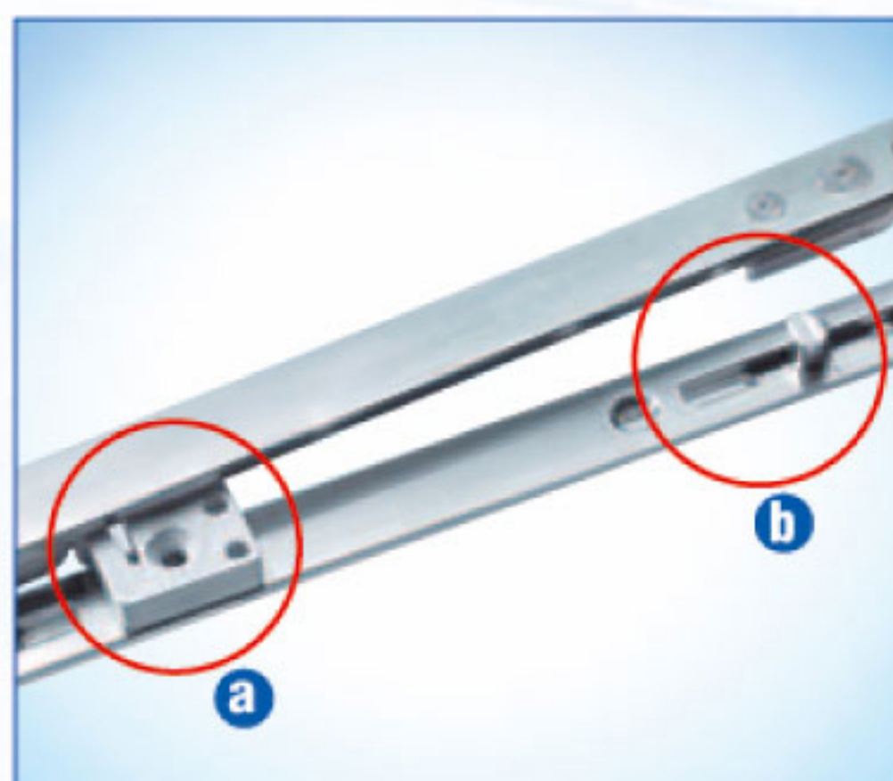
2 Est convenable L'entrebâilleur a optionnel b standard
